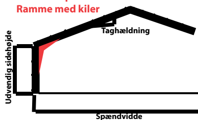
Standardspær Ramme med kiler
