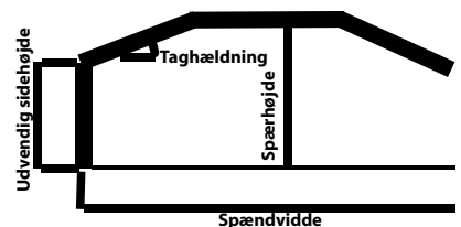
Indbygningsspær
